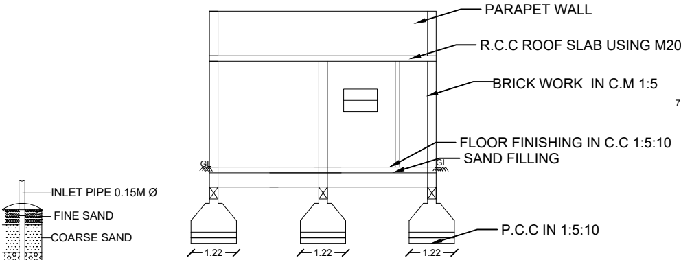
SECTION A-A
