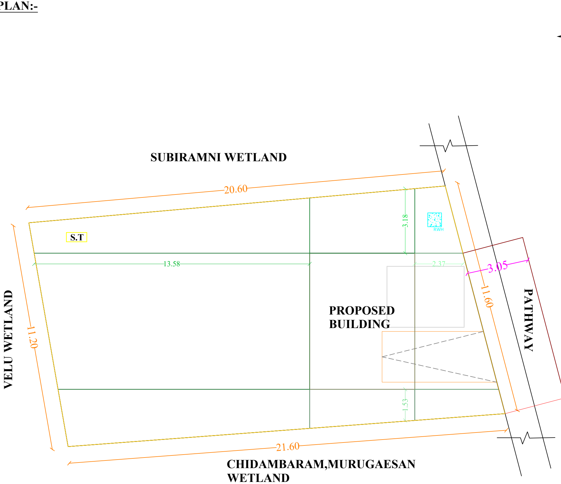
SITE PLAN:-
