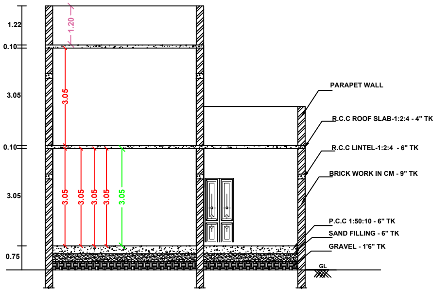
SECTION A-B
