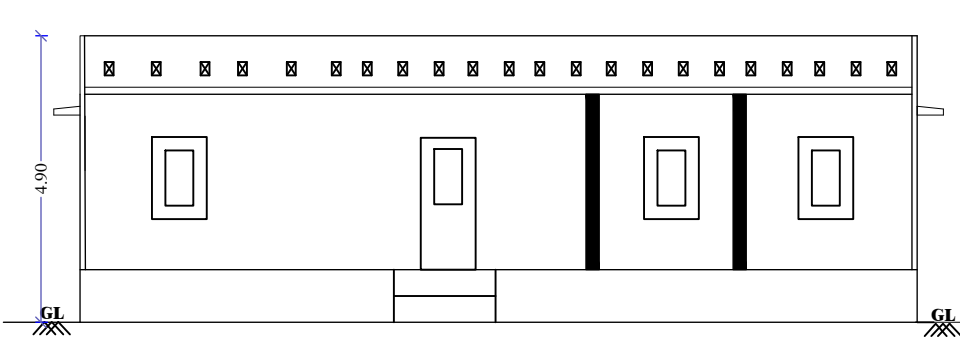
ELEVATION
