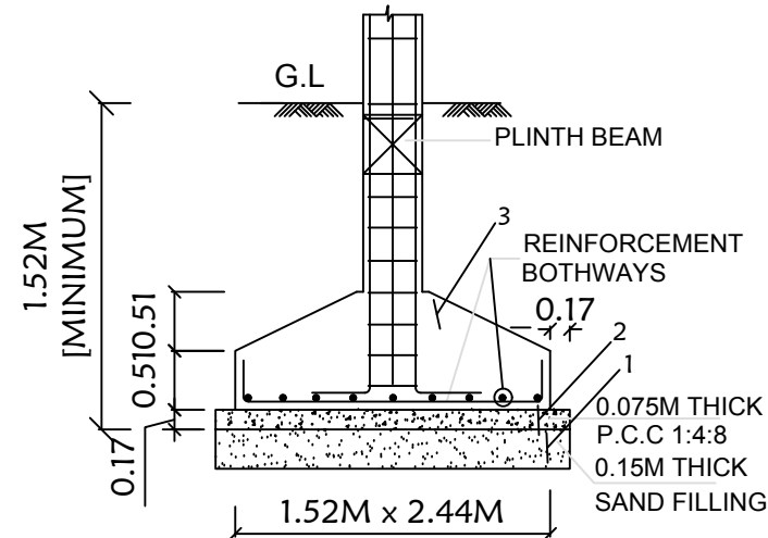
TYP. DET. COLUMN FOOTING
