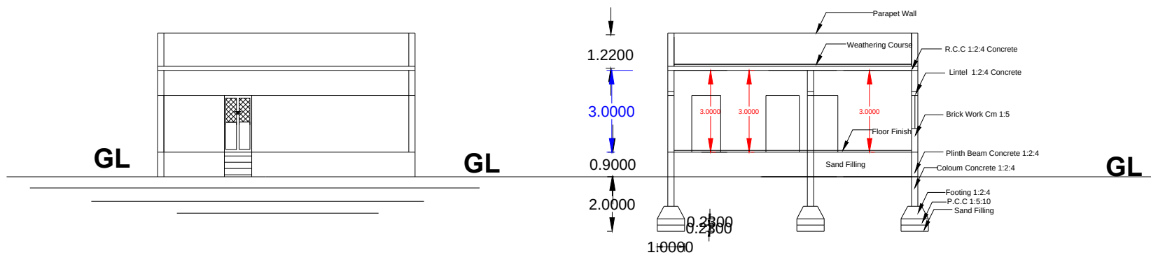
Elevation
