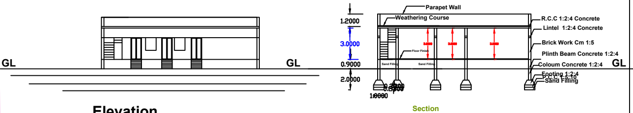
Elevation
