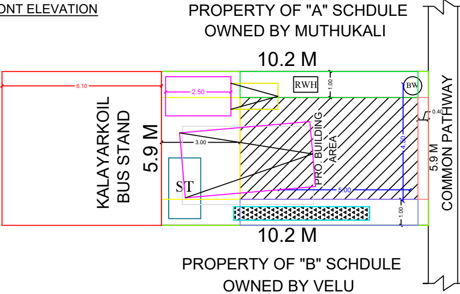
SITE PLAN(N.T.S)
