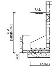
TYP. DET. CC
