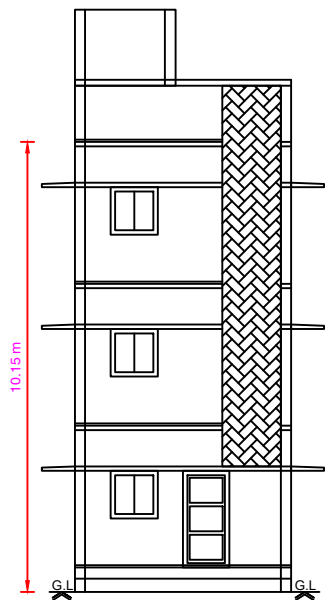
ELEVATION
