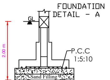
TYP. DET. COLUMN FOOTING
