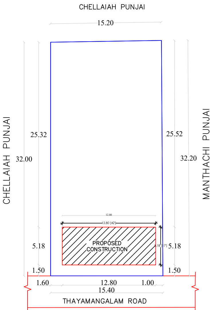
SITE PLAN (A2 - Scale : 1:120)
