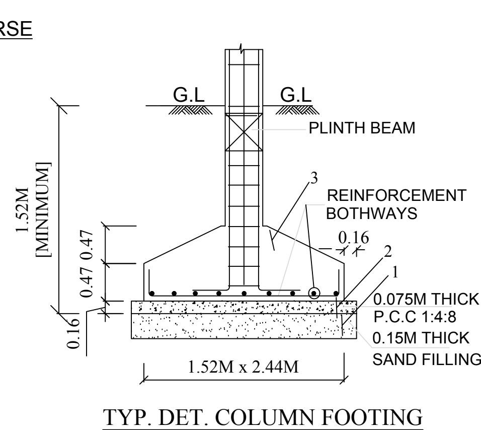
TYP. DET. COLUMN FOOTING
