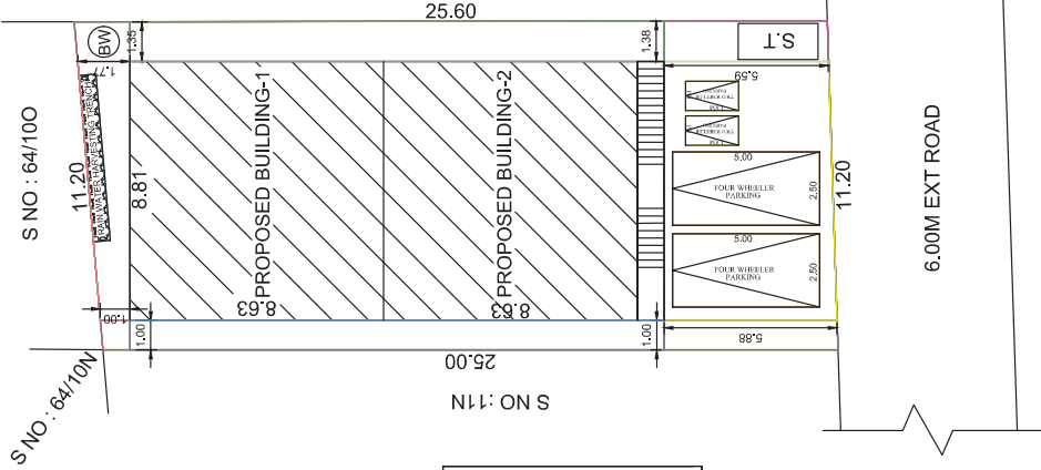
TOPO PLAN (SCALE - N.T.S)
