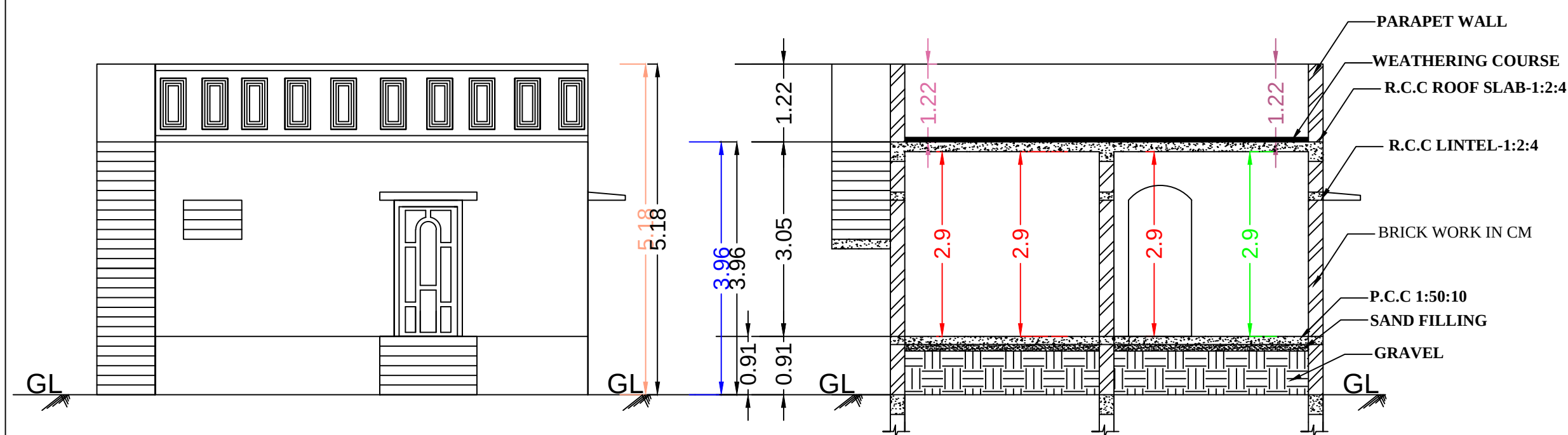
ELEVATION
