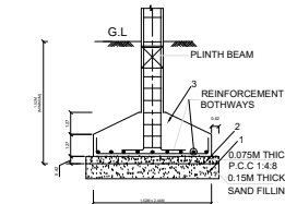
TYP. DET. COLUMN FOOTING
