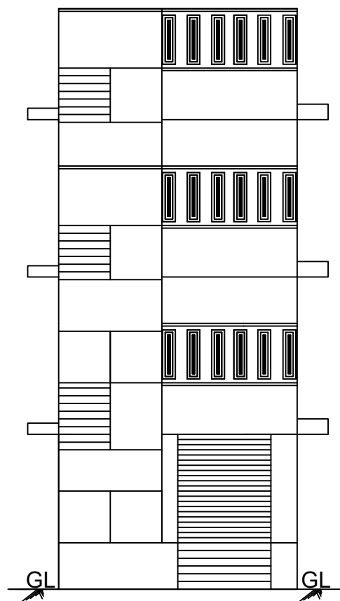
ELEVATION
