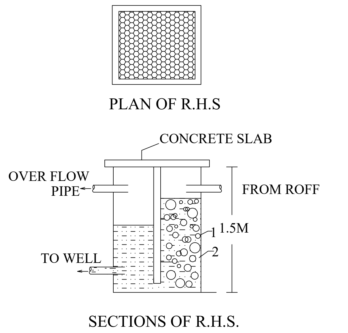
PLAN OF R.H.S
