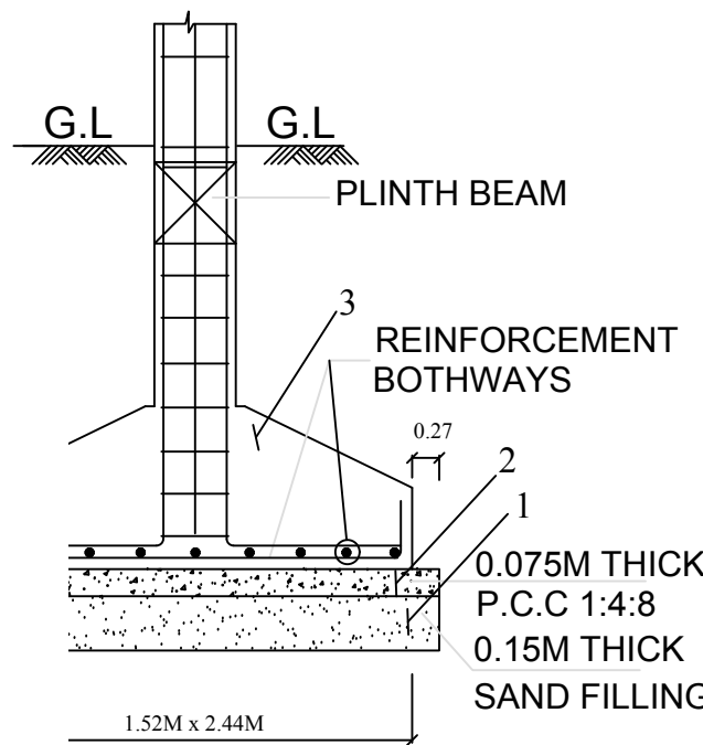
DET. COLUMN FOOTING
