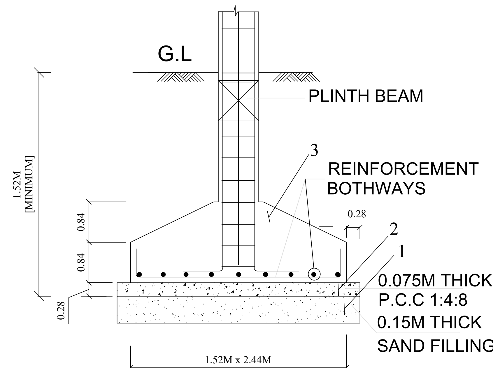
TYP. DET. COLUMN FOOTING
