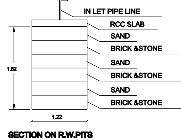
SECTION ON R.W.PITS
