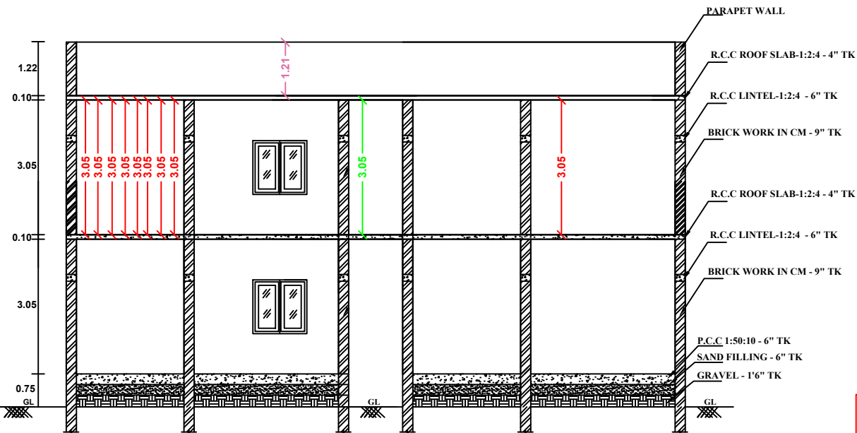
SECTION A-B
