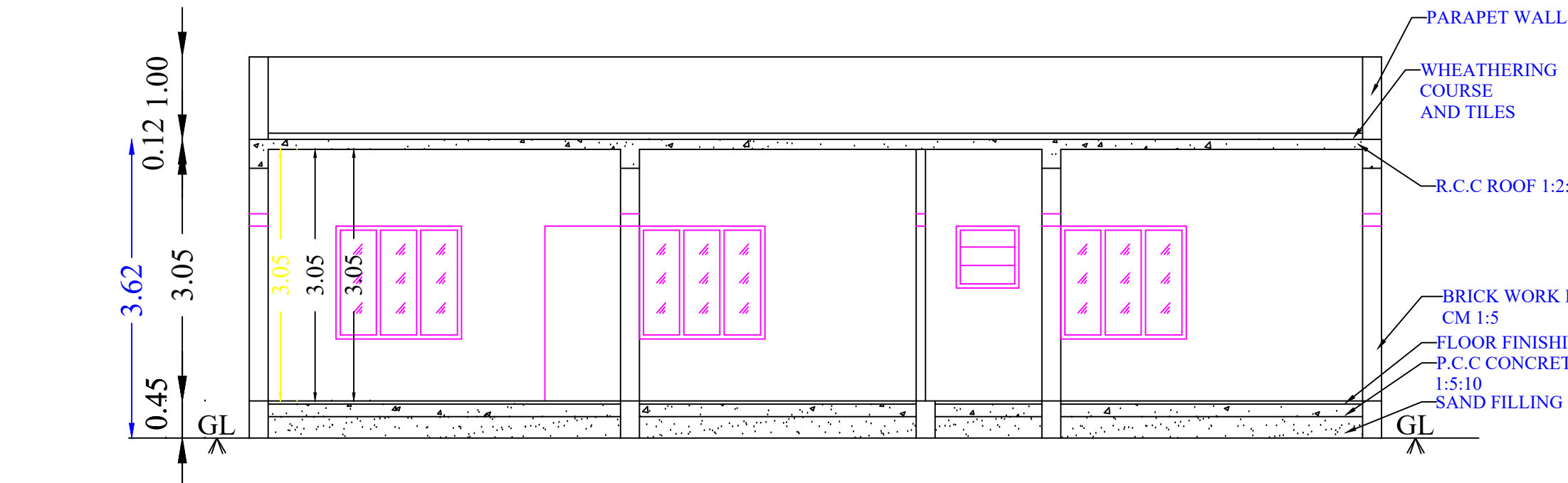
SECTION A-A
