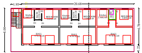
G. FLOOR PLAN
