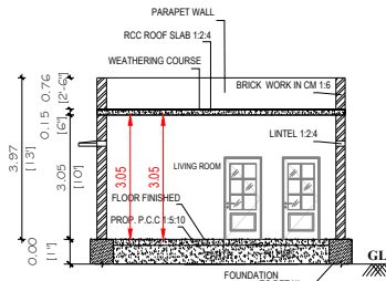
SECTION - 'AB'
