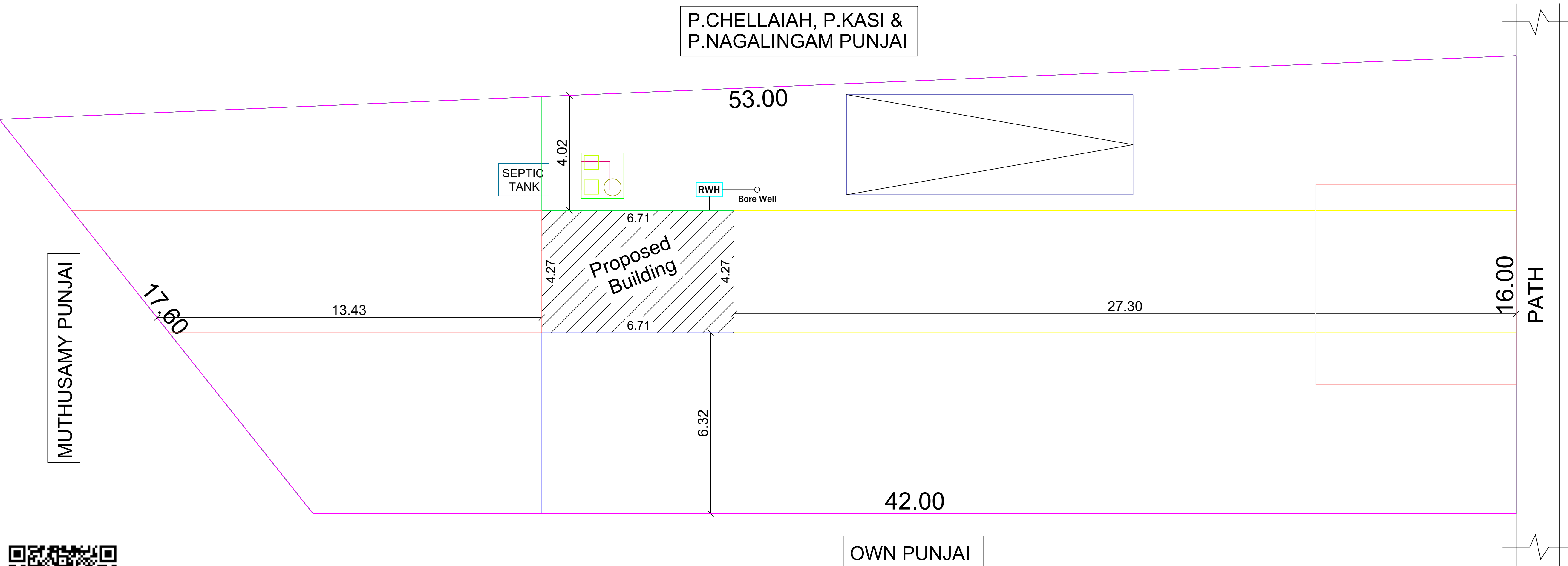
Site Plan Scale 1:100
