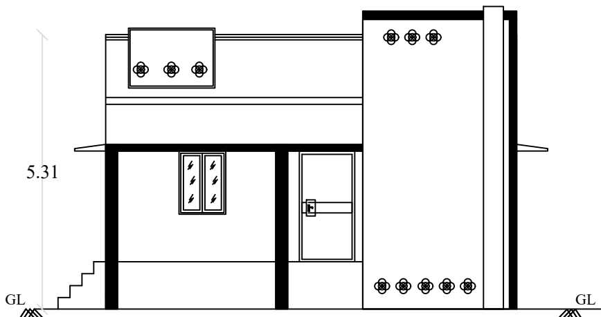
ELEVATION
