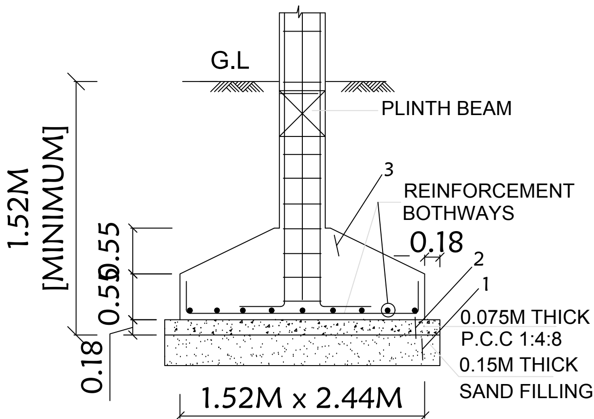
TYP. DET. COLUMN FOOTING
