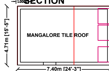
EX-BLK 2-PLAN
