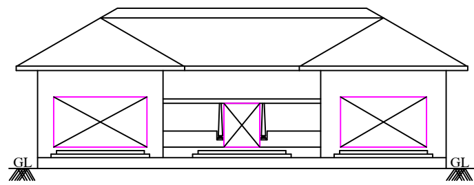
ELEVATION A-A
