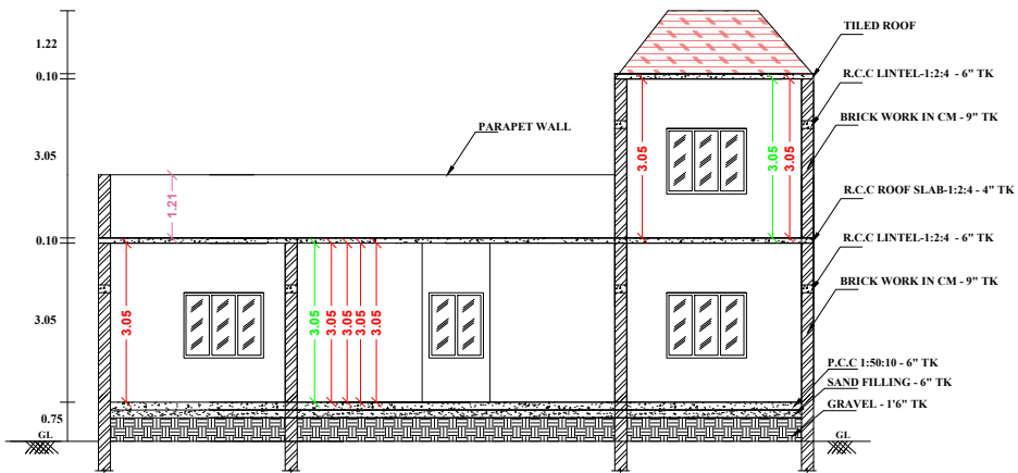
SECTION -AB
