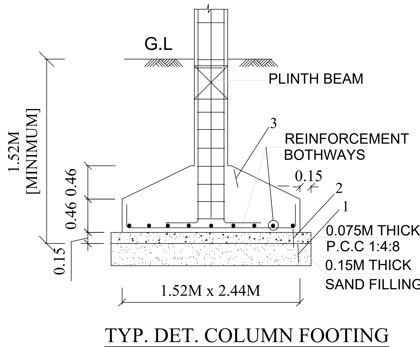
TYP. DET. COLUMN FOOTING
