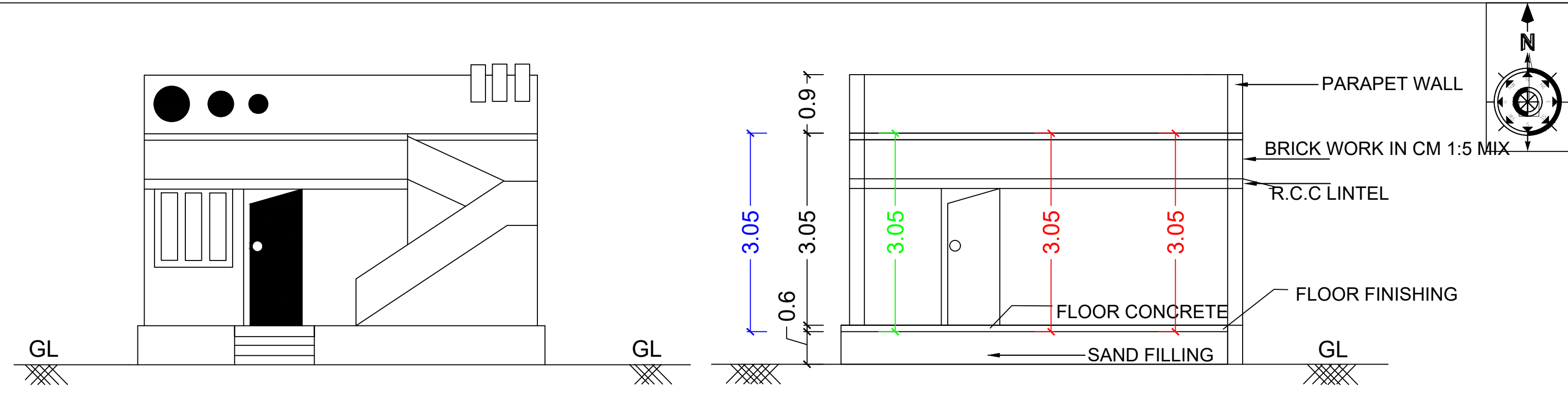
ELEVATION
