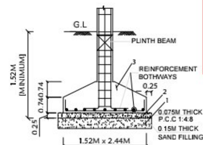
TYP. DET. COLUMN FOOTING
