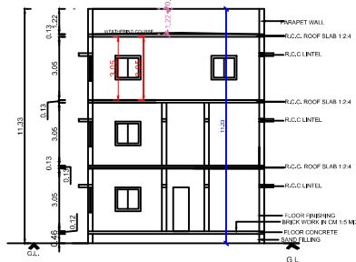
SECTION A-A1
