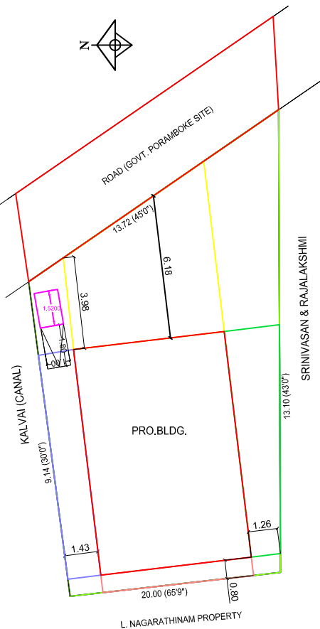
SITE PLAN 1 : 100
