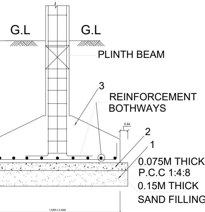
TYP. DET. COLUMN FOOTING
