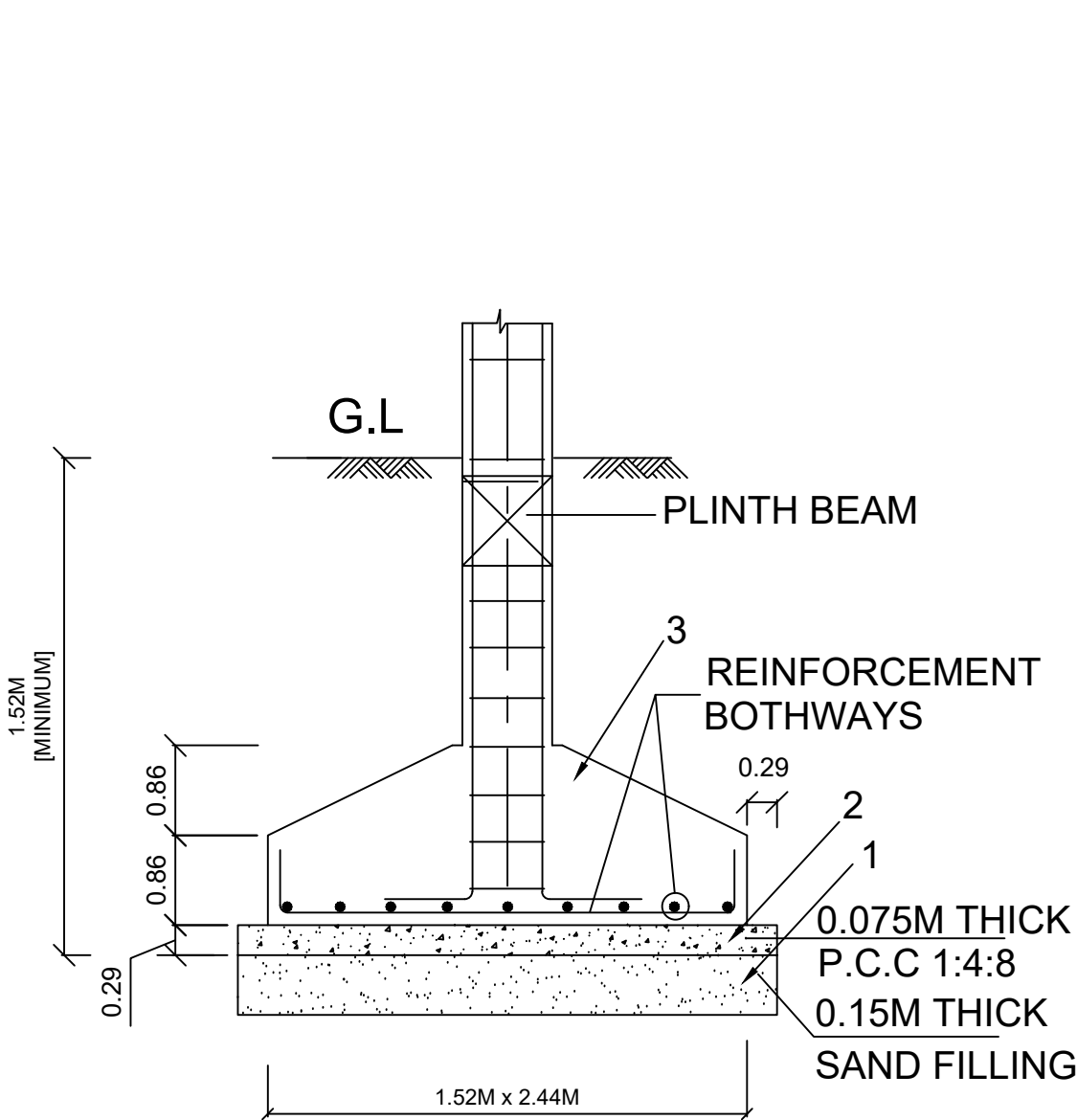
TYP. DET. COLUMN FOOTING
