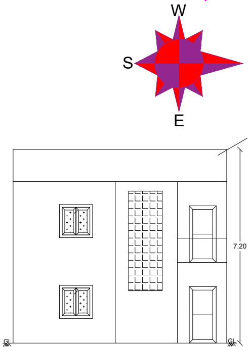
ELEVATION
