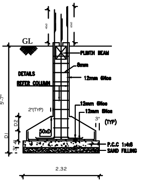
SCALE : 1:50.
