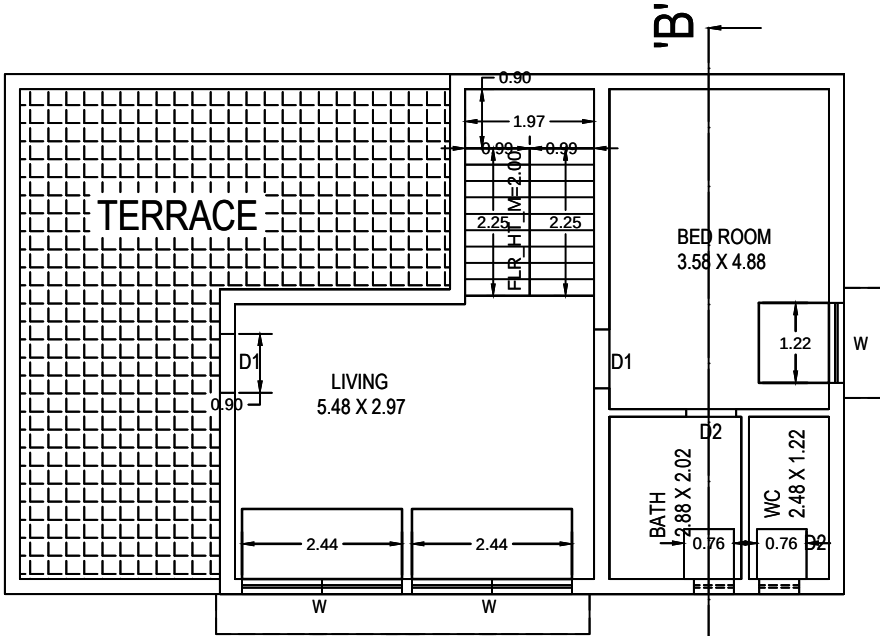
SCALE : 1:50.
