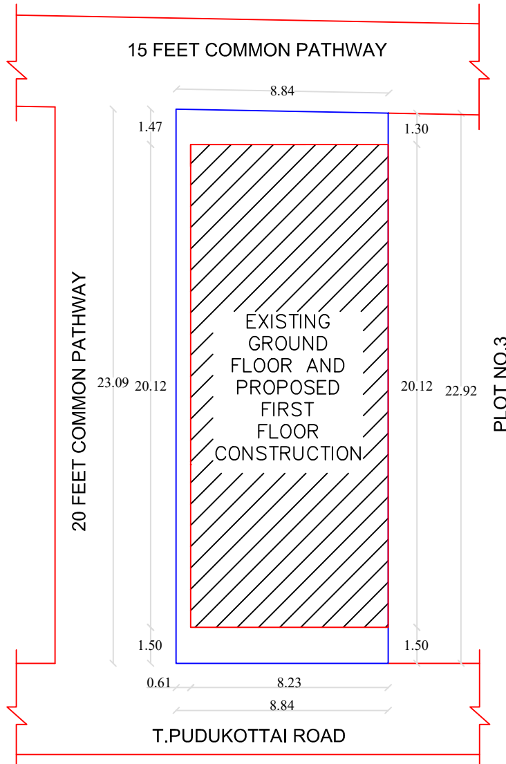
SITE PLAN (A2 - Scale : 1:350)
