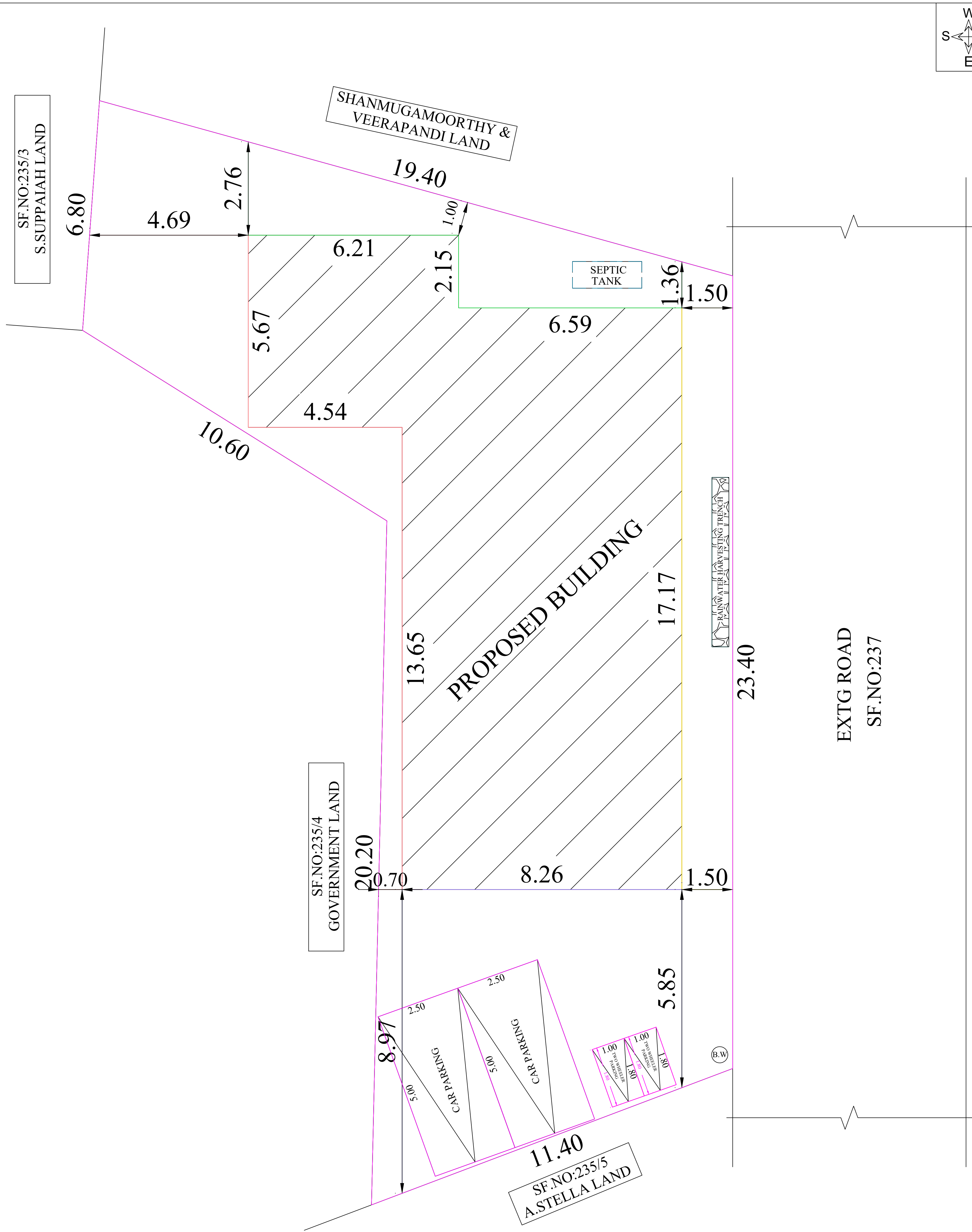
SITE PLAN 1:100
