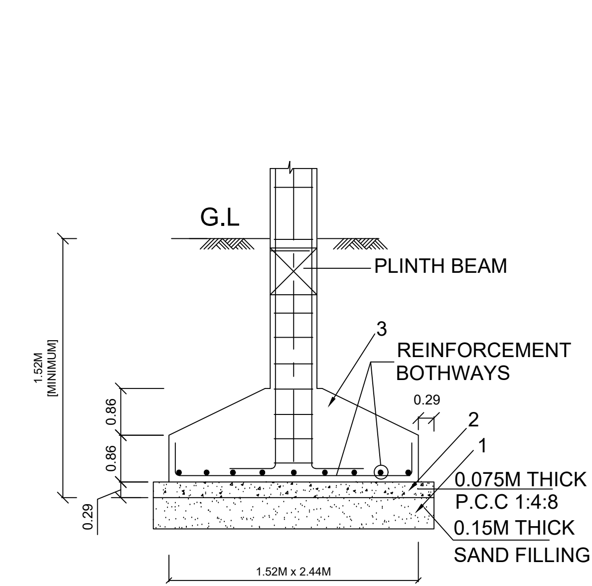
TYP. DET. COLUMN FOOTING
