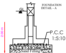
TYP. DET. COLUMN FOOTING
