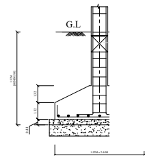
TYP. DET. COLUMN FOOTING
