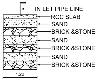
SECTION ON R.W.PITS
