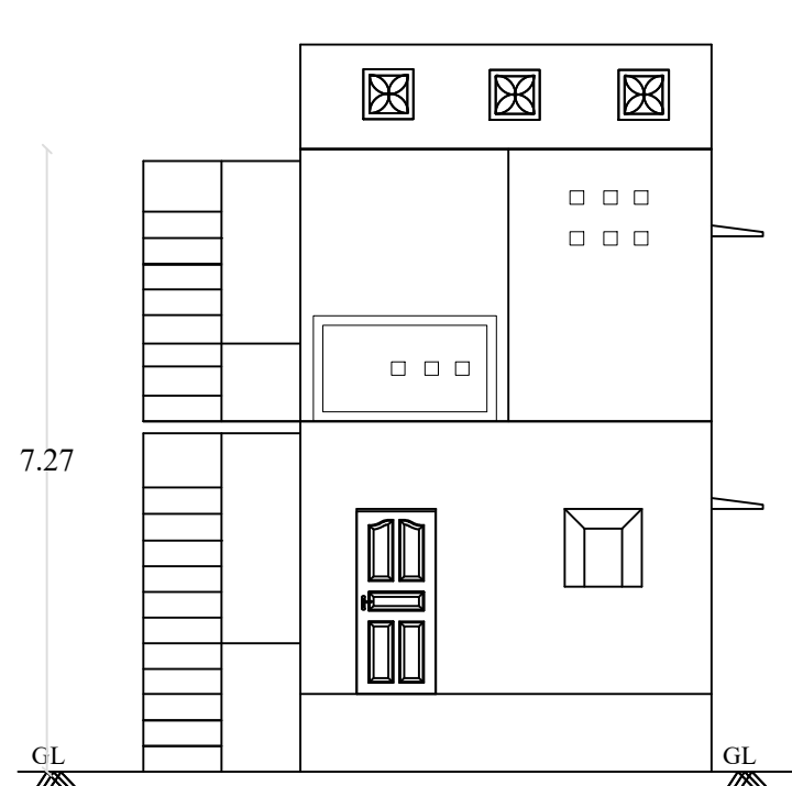
ELEVATION
