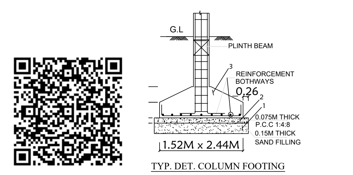
TYP. DET. COLUMN FOOTING
