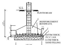
TYP. DET. COLUMN FOOTING
