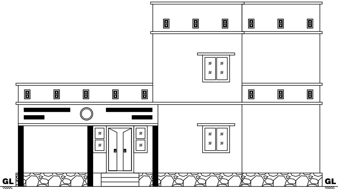
ELEVATION
